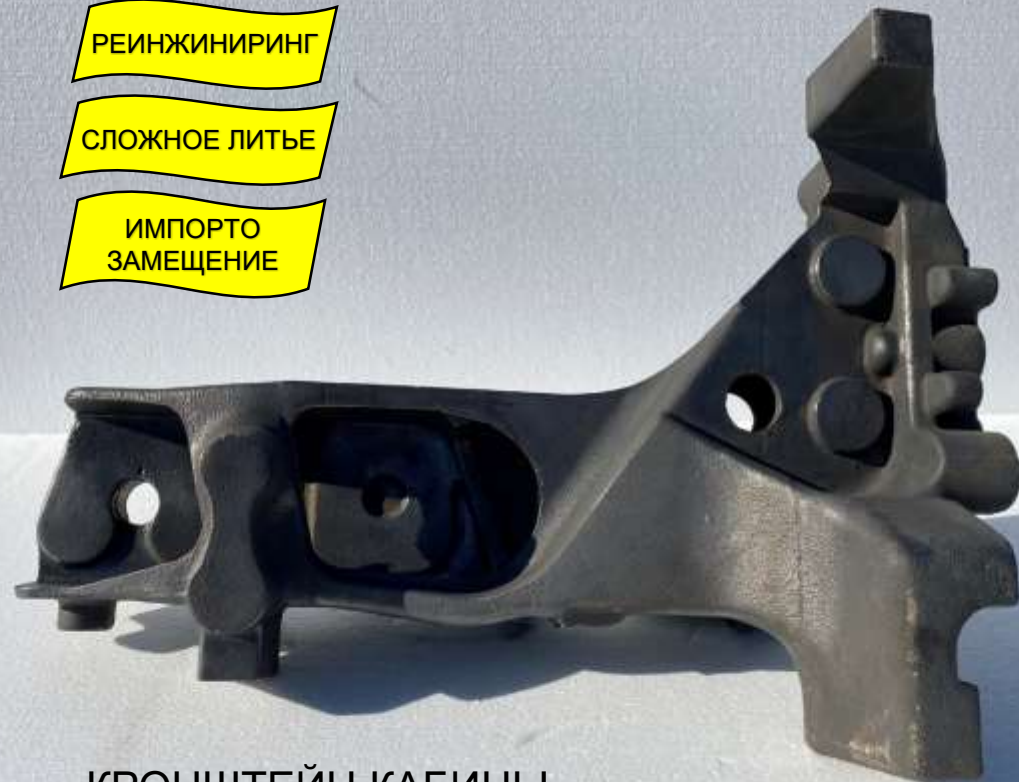
КРОНШТЕЙН КАБИНЫ полостная отливка ВЧ40 26,2 кг
